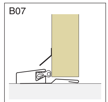
BUNDANSLAG INDADGÅENDE
