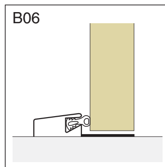
BUNDANSLAG UDADGÅENDE
