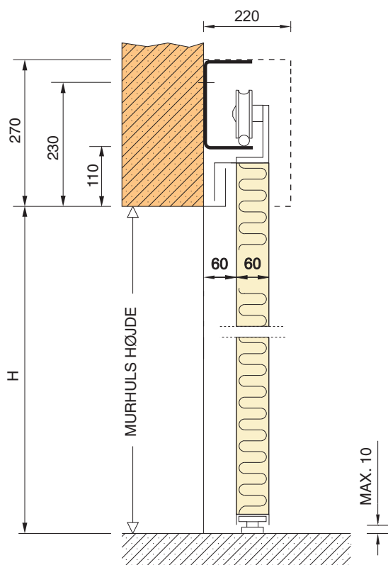
LODRET SNIT
