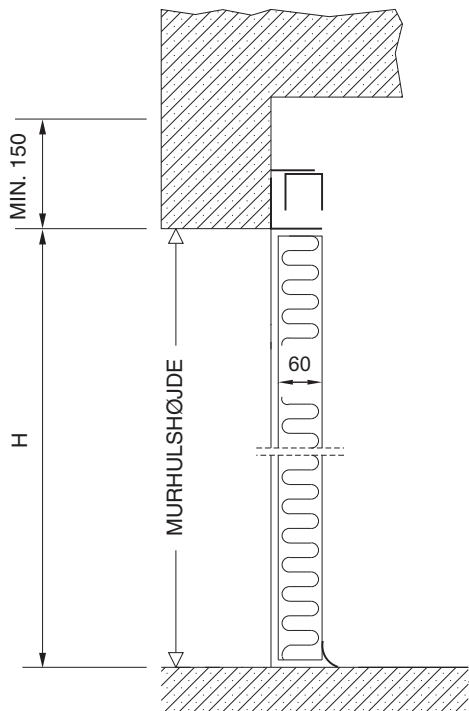
LODRET SNIT
