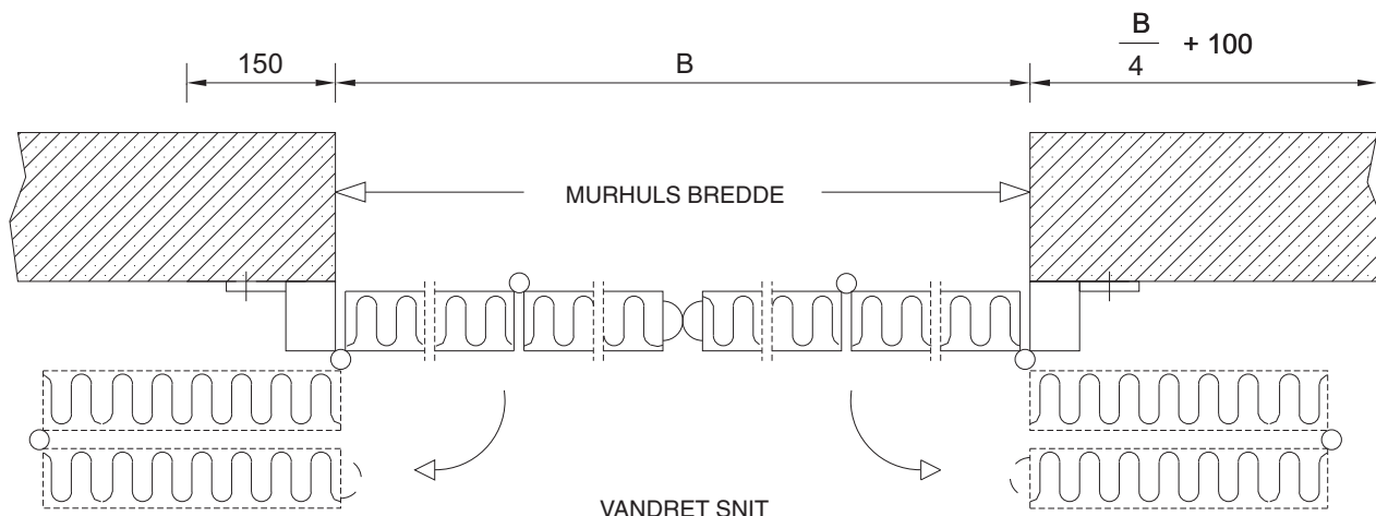
VANDRET SNIT
