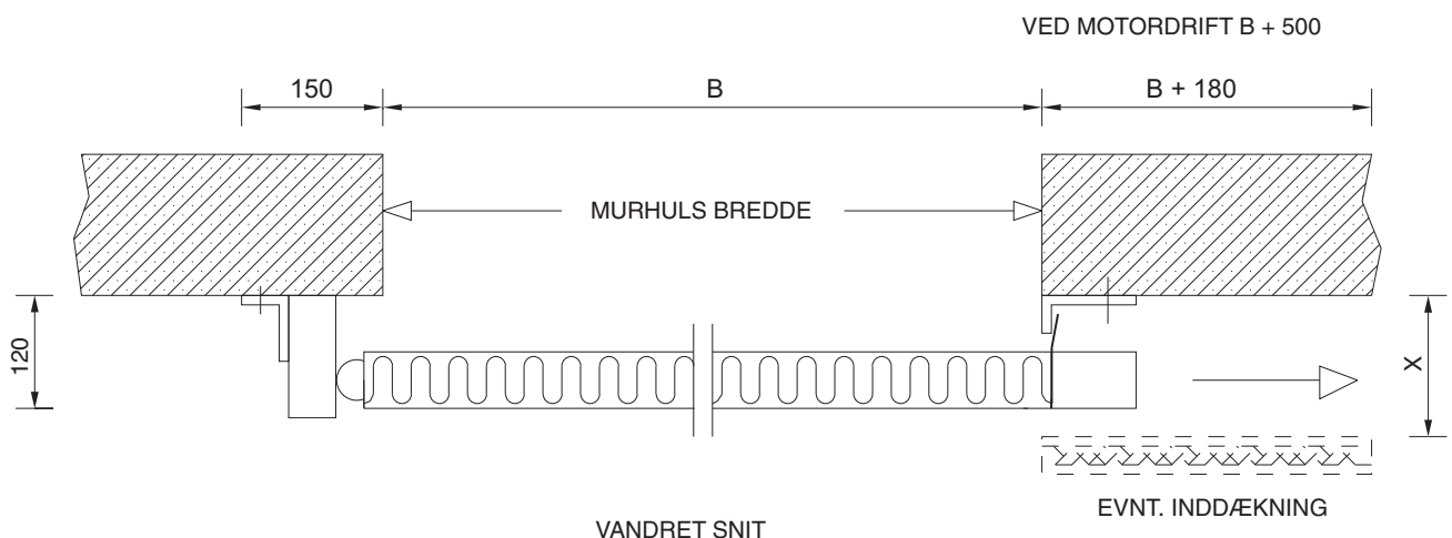
VANDRET SNIT
