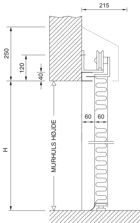
LODRET SNIT
