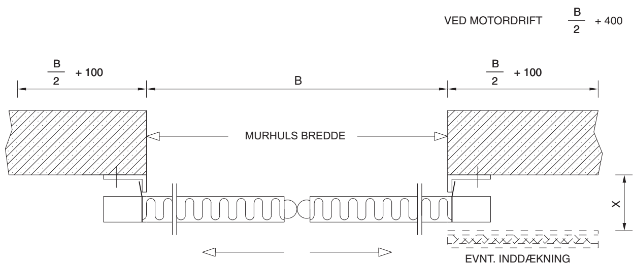
VANDRET SNIT
